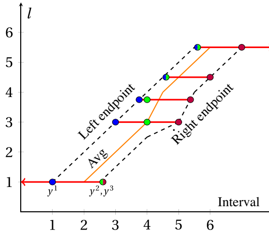
Fig. 2. The Y-Equilibria.
